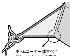
ボトムコーナー部すべてにシームシーリング剤を塗布してください。
